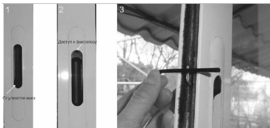
Регулировка фиксатора
